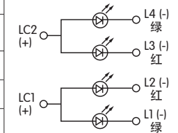
红 / 绿双色发光二极管
