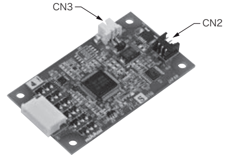
FT 控制板 FTCS05B 的更改示意图
